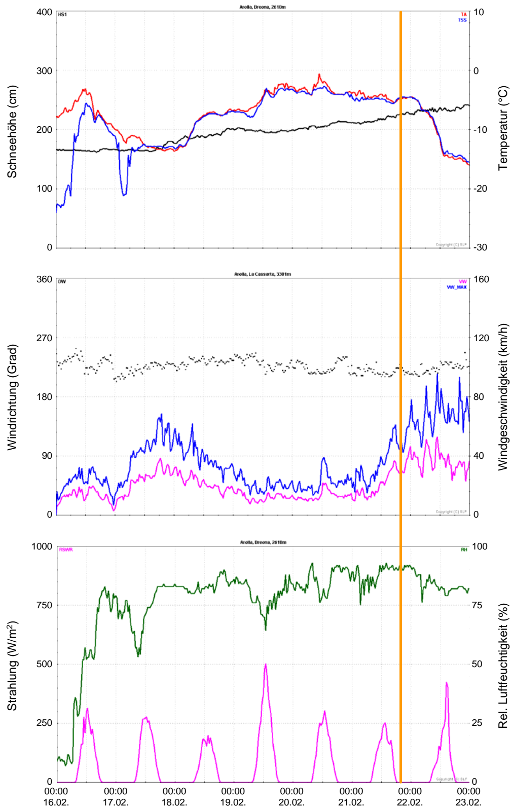
Abb. 2: IMIS-Messdaten der Station Bréona (ARO3) vom 16.-22. Februar 1999. Schneehöhe, Luft- und Schneeoberflächentemperatur (oben), Windrichtung und -geschwindigkeit (Mittel und Böenspitzen) gemessen an der Gipfelstation La Cassorte (3301 m ü.M.) (ARO1) (mitte), und relative Luftfeuchtigkeit und Strahlung (unten). Die orange Linie bezeichnet den ungefähren Zeitpunkt des Lawinenabganges.
