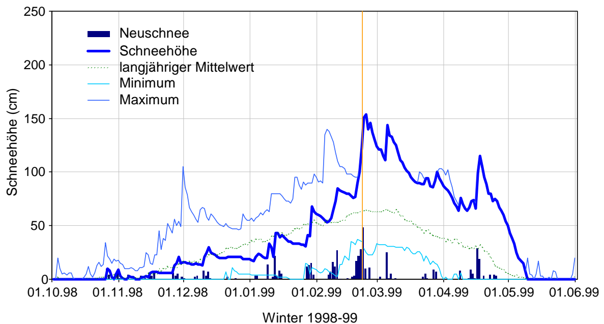
Abb. 1: Schneehöhenverlauf (im Vergleich mit den langjährigen Werten) und Neuschneemenge an der SLF Vergleichsstation Arolla 1890 m ü. M. Die orange vertikale Linie bezeichnet den Zeitpunkt des Lawinenabganges von Evolène.
