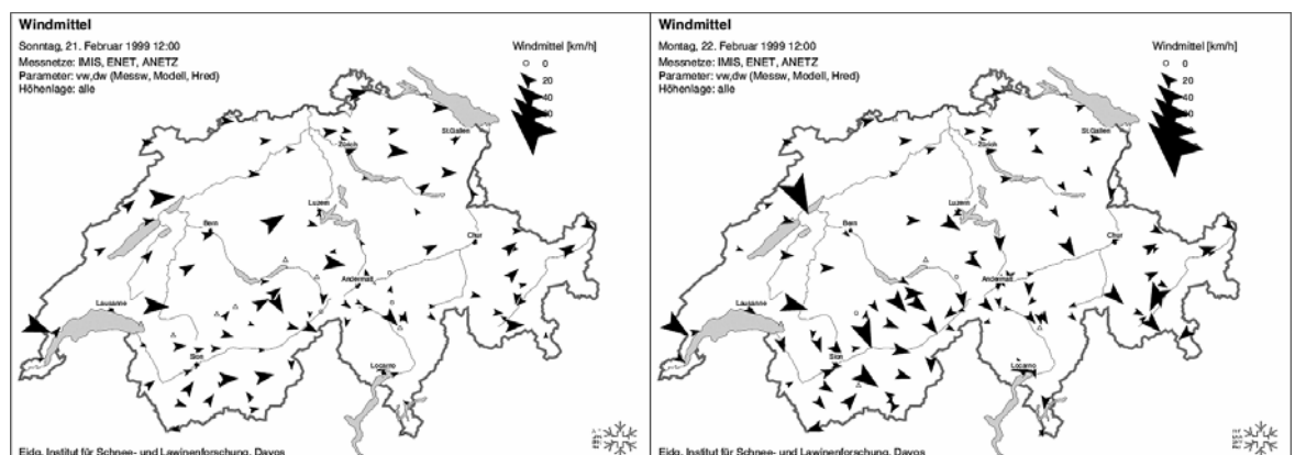
Abb. 3: Windrichtungen in der Schweiz am 21. Februar 1999, mittags (links) und am 22. Februar 1999, mittags (rechts).
