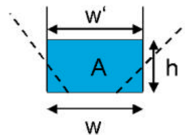
Abbildung 51: Runsens – Gemittelte FlieSSbreite mit rechtwinkligen Seiten.
