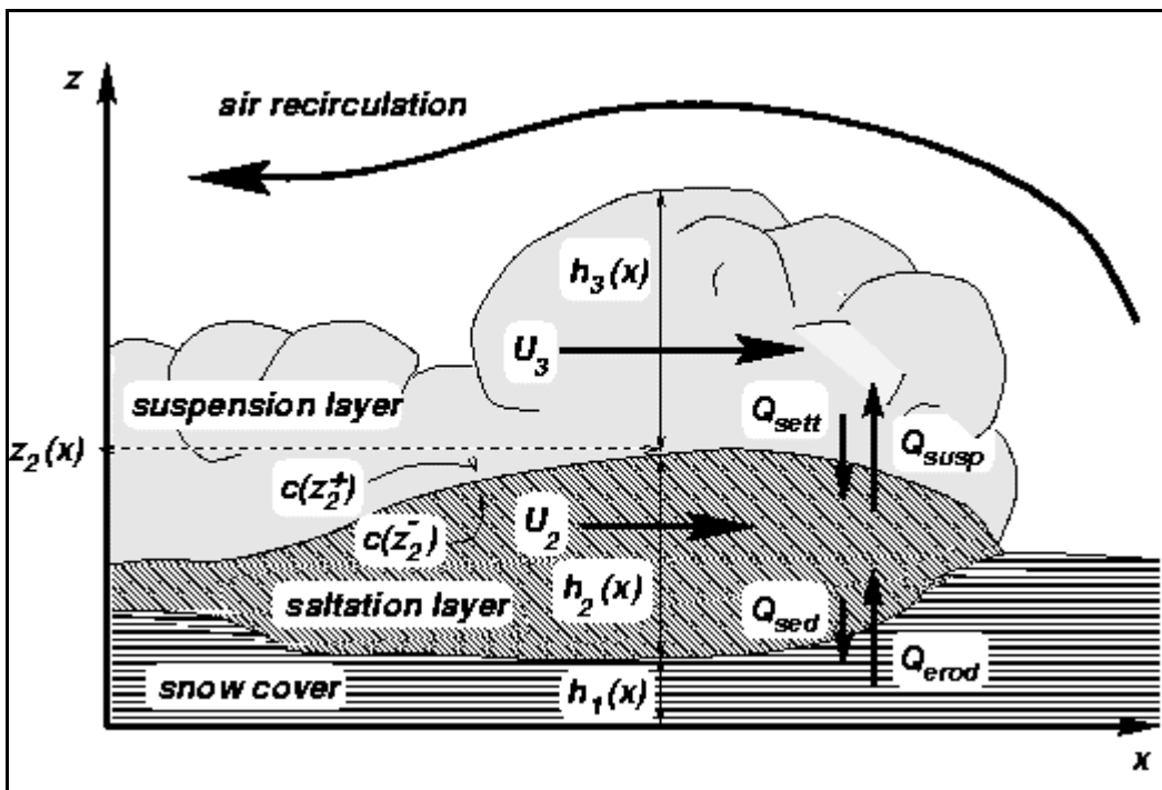
Abbildung 43: Schematische Darstellung einer Staublawine.
