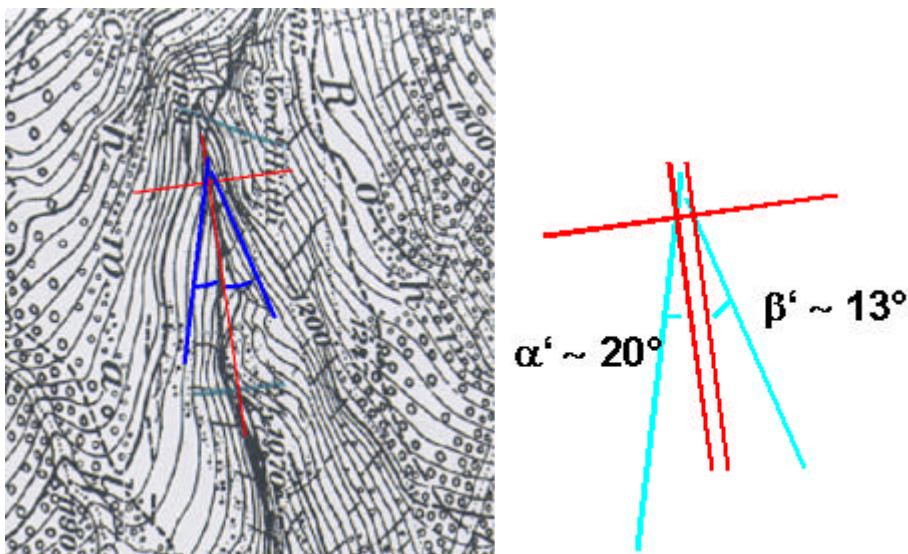
Abbildung 53: Höhenlinienwinkel aus einer Karte gelesen. Die Hangneigung beträgt 22.6°.
