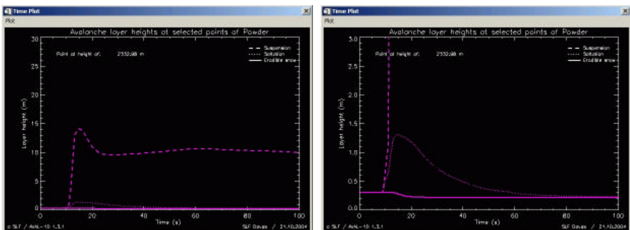
Abbildung 48: Schneehöhen Time Plot ; links -> praktisch nur Suspensionshöhe, rechts -> skaliert auf 3m, Saltations- und erodierbare Schneehöhe ablesbar.
