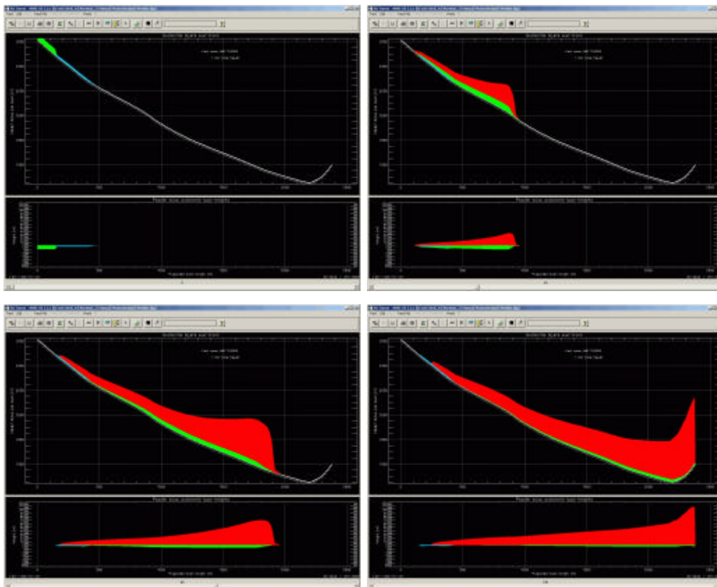
Abbildung 44: Animation der Vallée de la Sionne Staublawine.
