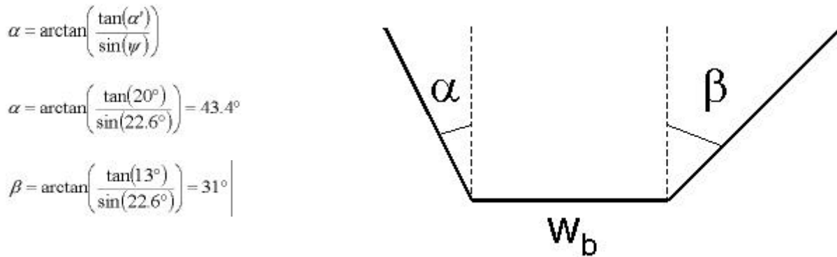
Abbildung 54: Umrechnung der Höhenlinienwinkel in effektive Profil-Winkel.
