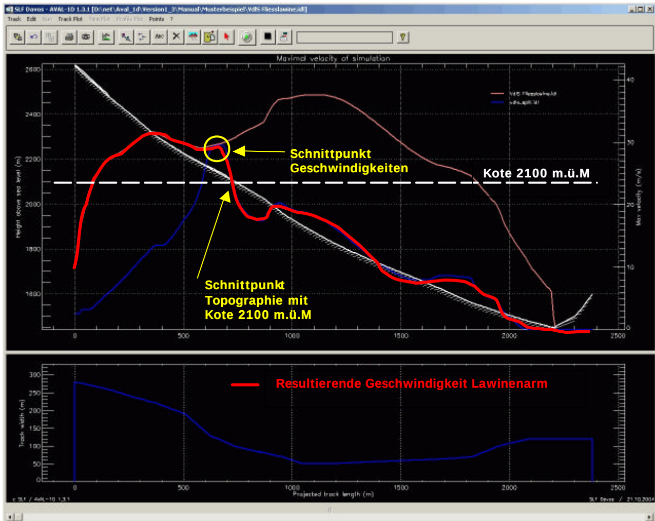
Abbildung 40: Überlagerung der Ursprungs-Simulation mit der gesplitteten Simulation; dargestellt ist die max Geschwindigkeit.
