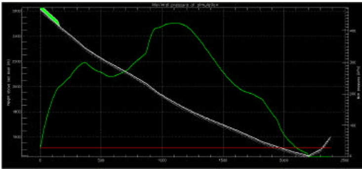
Abbildung 34: Track Plot: Maximale Schneehöhe (blau), maximale Geschwindigkeit (rot) und maximaler Druck (grün, von oben nach unten).
