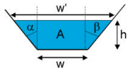
Abbildung 52: Runsens – Talbodenbreite und variable Seitenwinkel entlang der Lawinenbahn.
