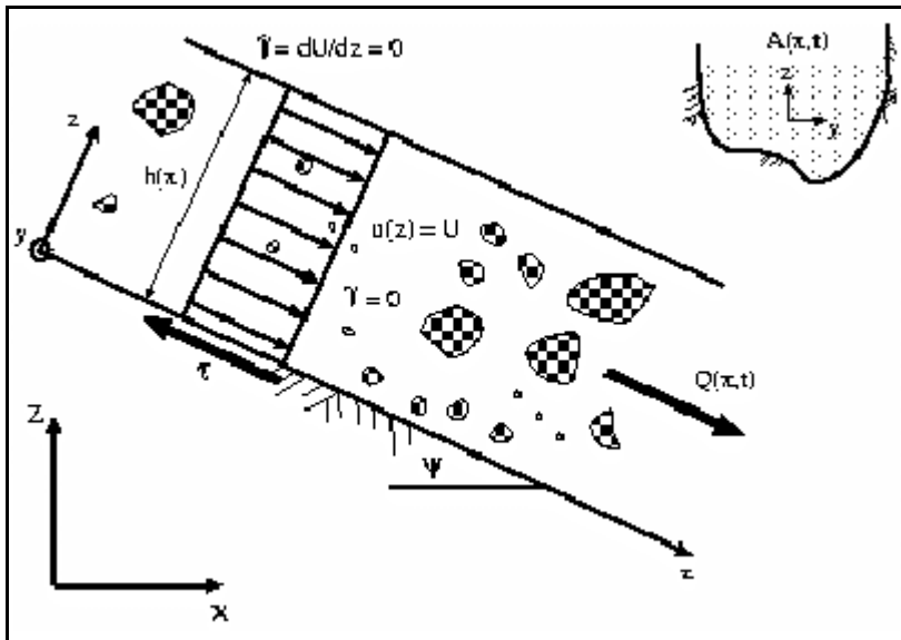
Abbildung 32: Schematische Darstellung einer Fliesslawine.
