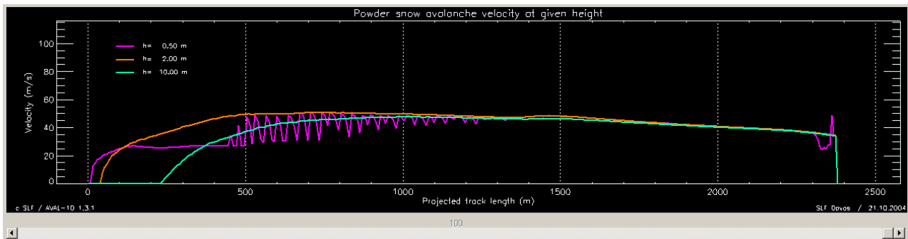
Abbildung 47: Maximale Werte der Geschwindigkeit in drei verschiedenen Höhen ab Boden, 0.5m, 2m und 10m.
