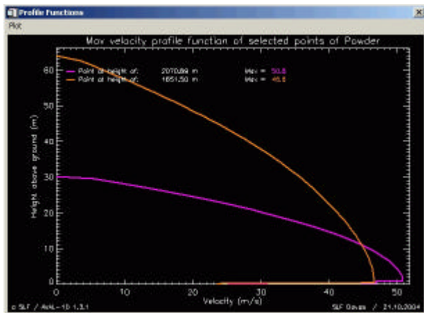
Abbildung 49: Geschwindigkeits Profile Plot für zwei Punkte.
